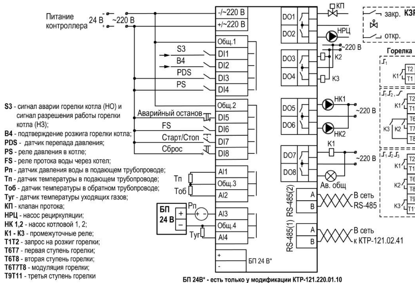
Рисунок 7.4 – Схема подключения
