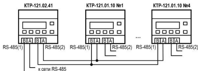
Рисунок 5.1 – Соединение каскадного регулятора с котловыми
