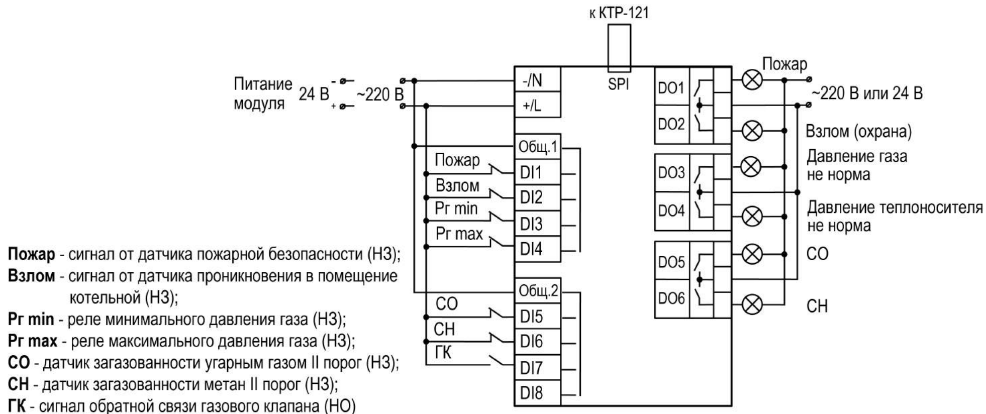
Рисунок 7.5 – Схема подключения к ПРМ сигналов общекотельных аварий
