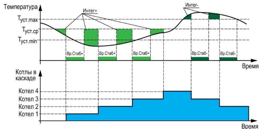
Рисунок 10.2 – Регулирование температуры
