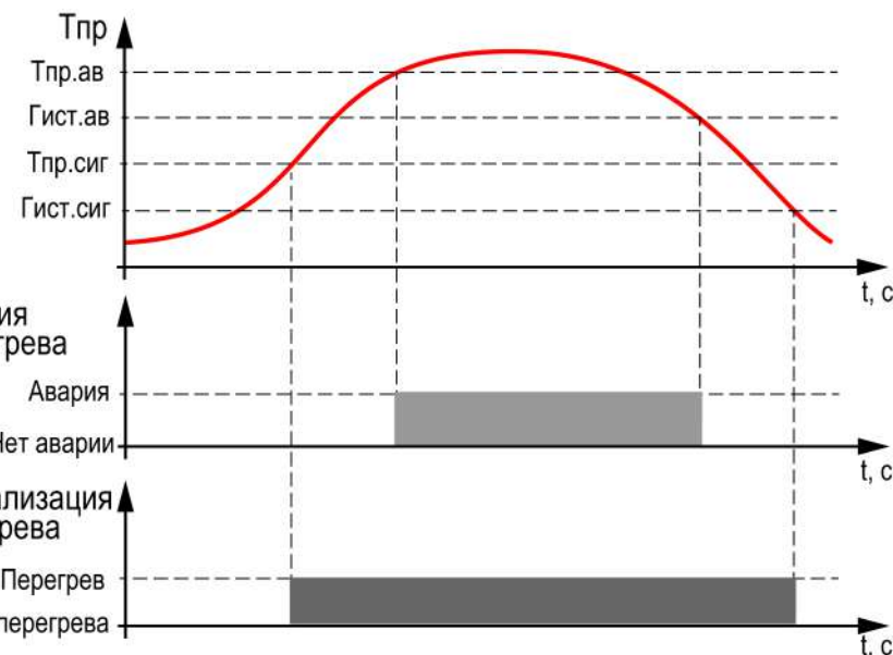
Рисунок 10.6 – Принцип определения и сброса аварии и сигнализации перегрева
