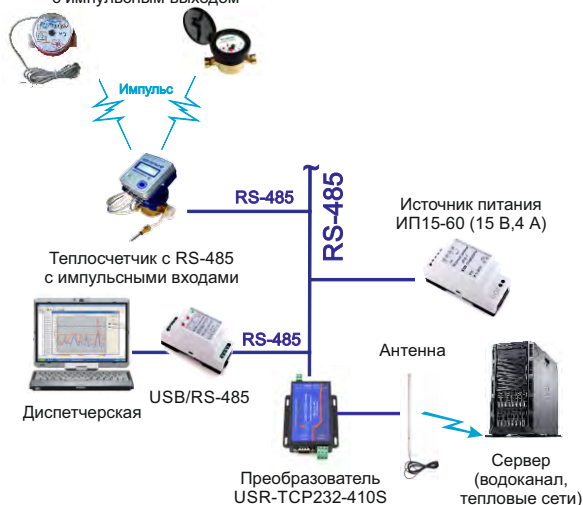
Счетчик холодной и горячей воды ПУЛЬСАР с импульсным выходом
