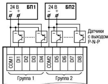
Рисунок 5.8 – Схема подключения датчиков с выходным транзистором р-п-р-типа
